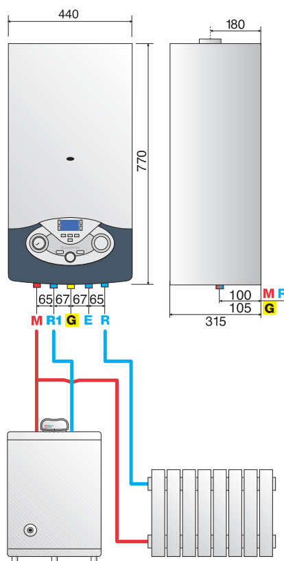
Ejemplo de instalación con acumulador para producción de ACS.
